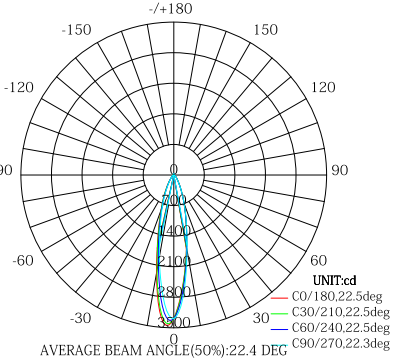
20°(Symmetric)
